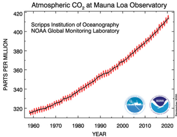
Abbildung 5 | Gemessene Konzentration der globalen CO 2 -Konzentration in der Troposphäre (Quelle NOAA 2021; http://www.esrl.noaa.gov/gmd/ccgg/trends/ ).
